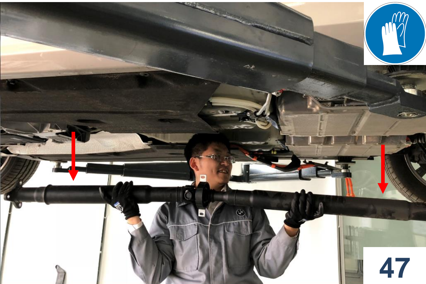
BMW 530Le
